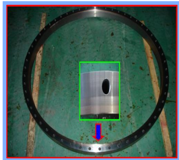
Clad Flange
